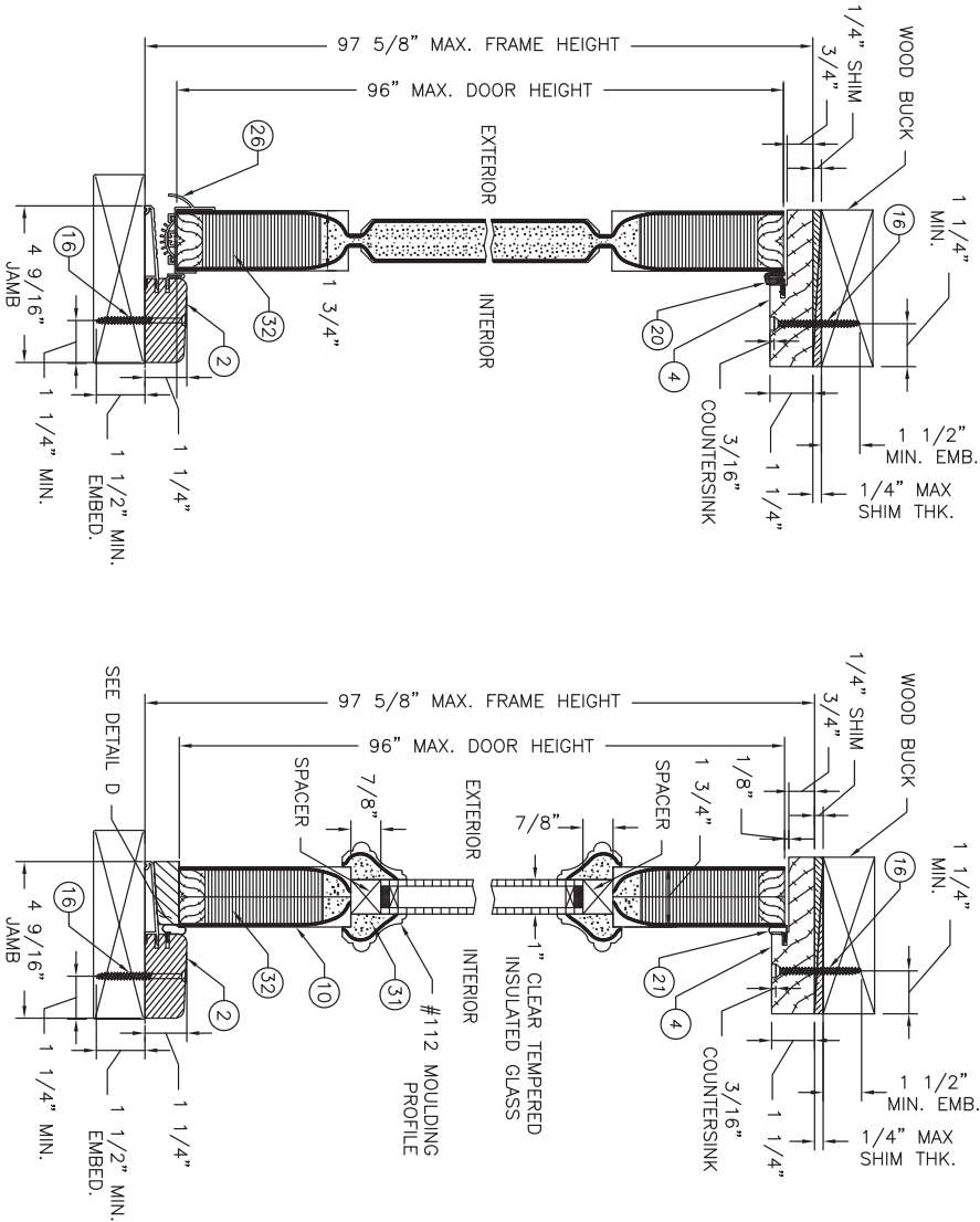
1 VERTICAL CROSS SECTION TYP DOOR SCALE: 3\"/>
